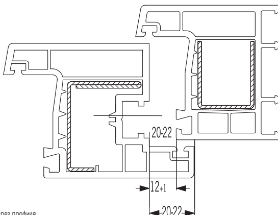
Рис. 1: Разрез профиля
