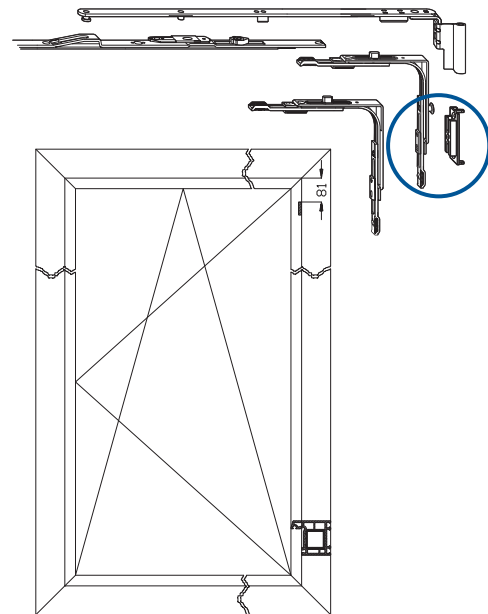
Размеры для монтажа ответных частей даны при фальцевом зазоре 12 мм.
